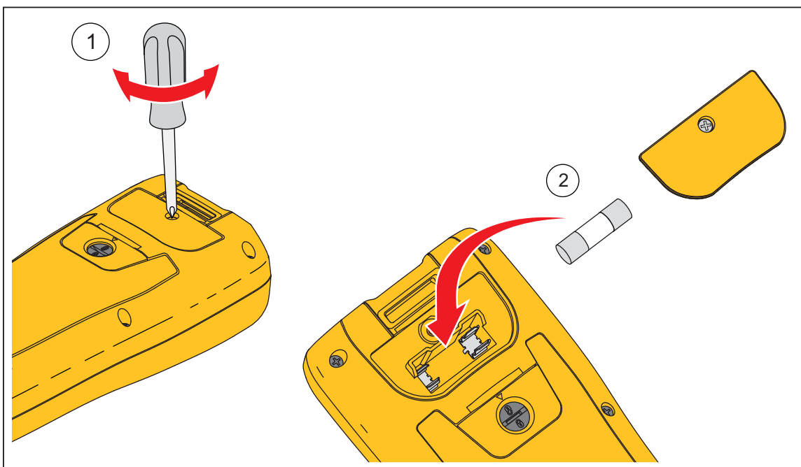
Figura 6-2. Substituição do fusível
