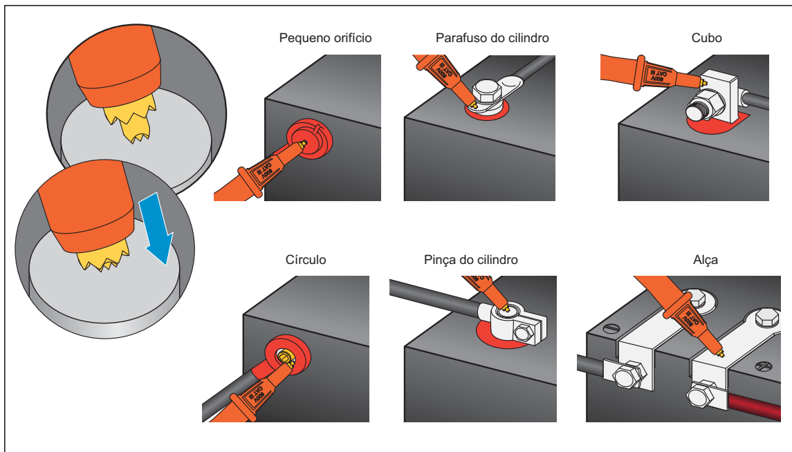
Figura 3-2. Conectar a ponta de prova na bateria
