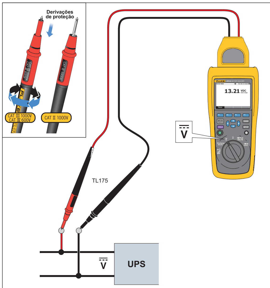
Figura 3-5. Medir tensão CC com o TL175
