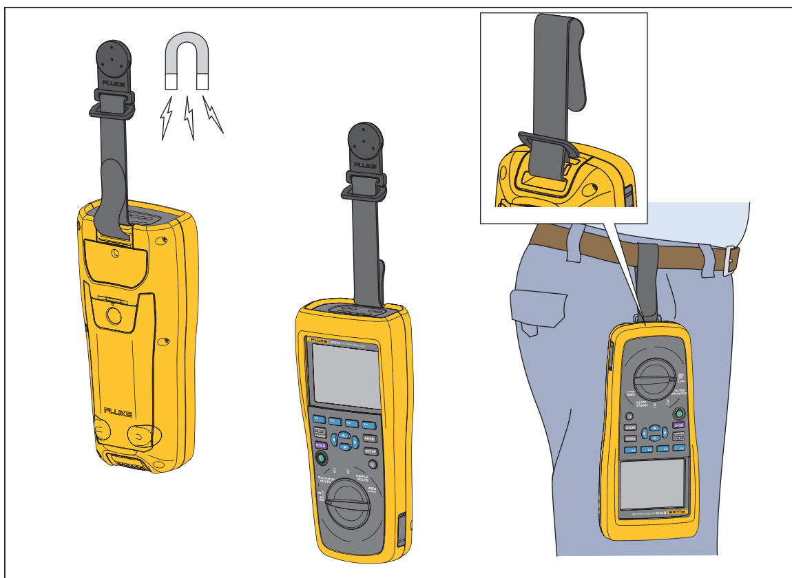
Figura 2-2. O cinto
