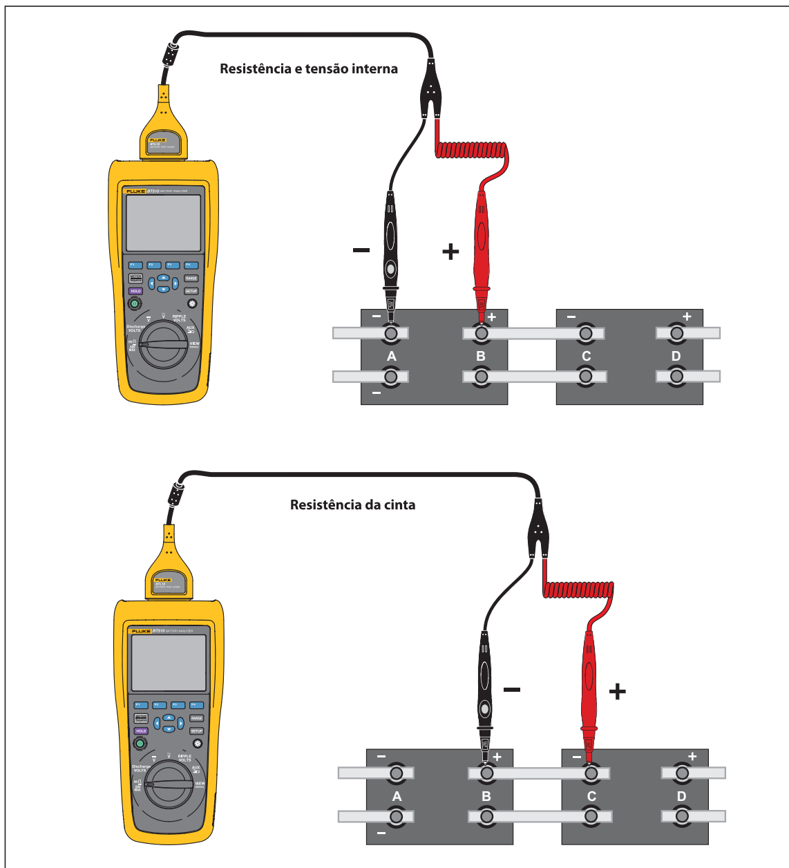
Figura 3-1. Testar a tensão e resistência interna da bateria ou a resistência da cinta
