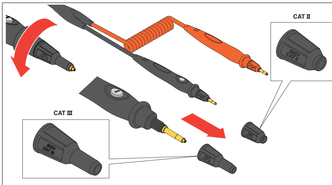
Figura 6-3. Substituir as pontas da sonda
