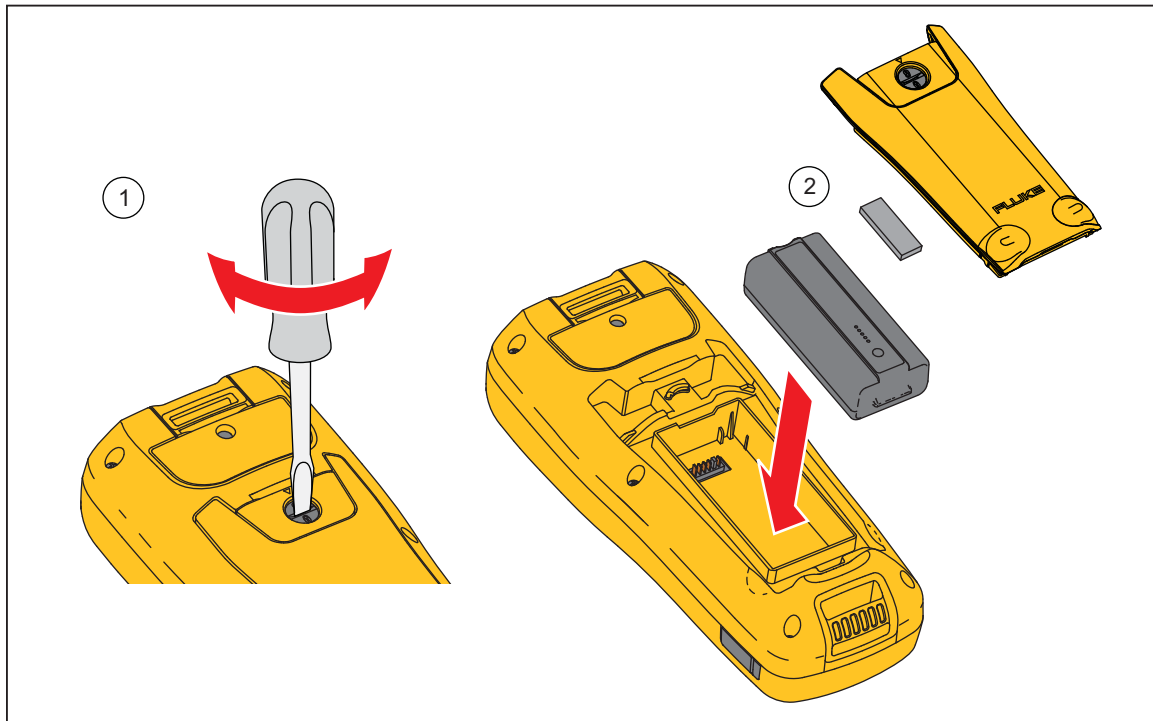
Figura 6-1. Instalar ou substituir um pacote de baterias
